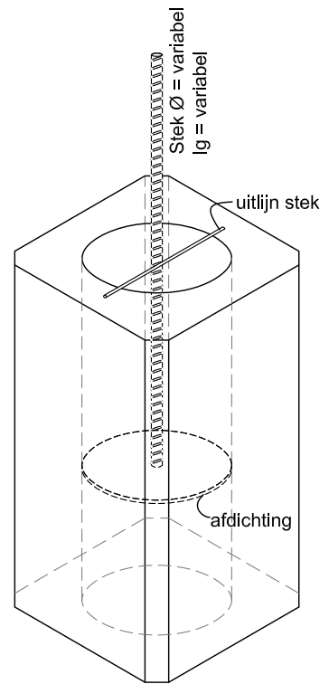
Isometrie - bovenste paal gedeelte
