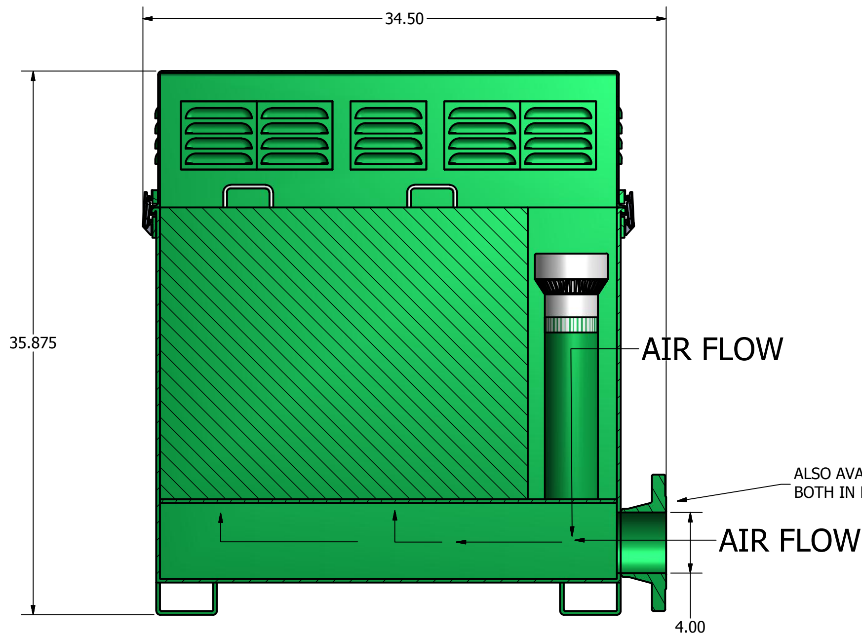
SECTION A-A SCALE 0.16 : 1
